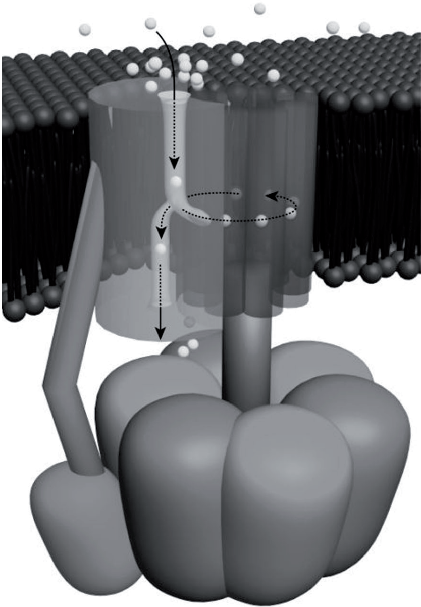
(Рисунок 1) Подпись: F 0 /F 1 -АТФсинтаза
