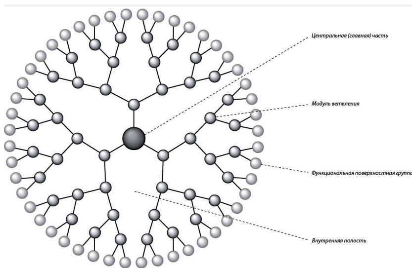
Рисунок 2 “Незагруженный” дендример.
